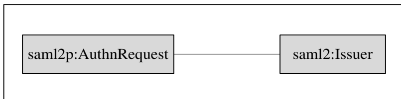
Рисунок 7 – Структура AuthnRequest
