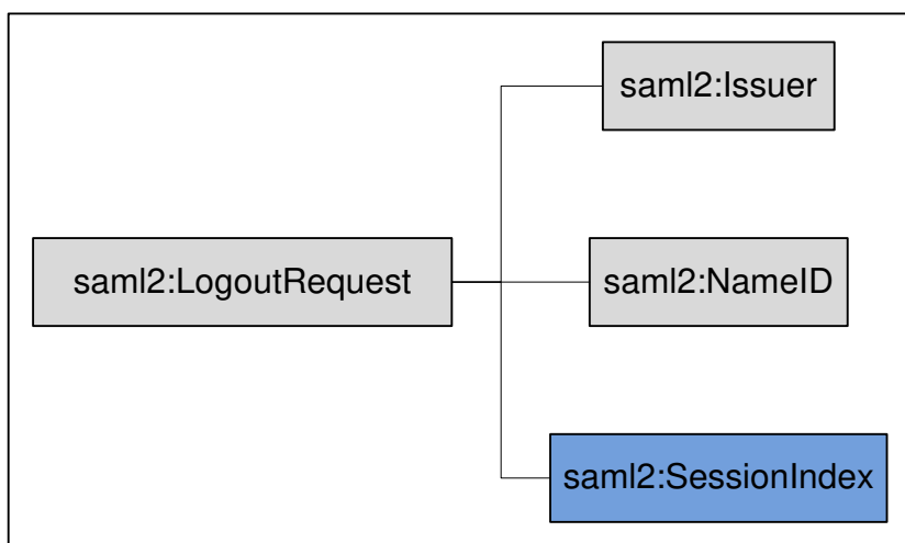
Рисунок 11 – Структура LogoutRequest
