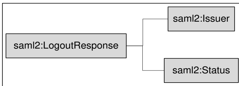
Рисунок 12 – Структура LogoutResponse
