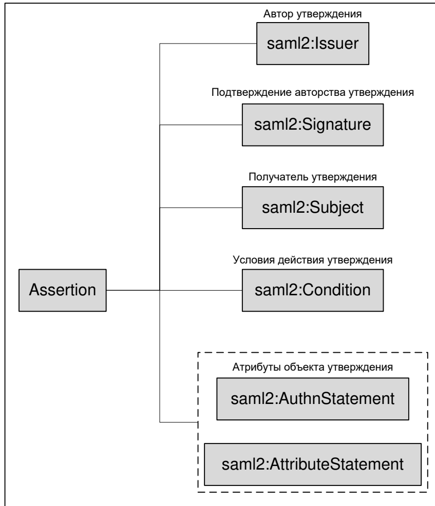
Рисунок 8 – Структура AuthnResponse
